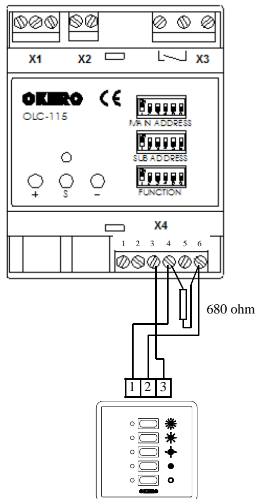
Figur 3. Inkopplin av DML panel.
